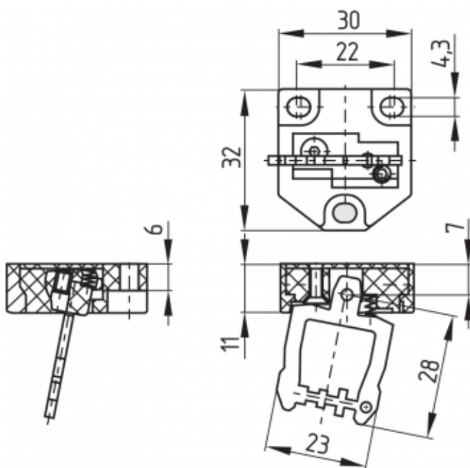
Flexible actuator B6L
