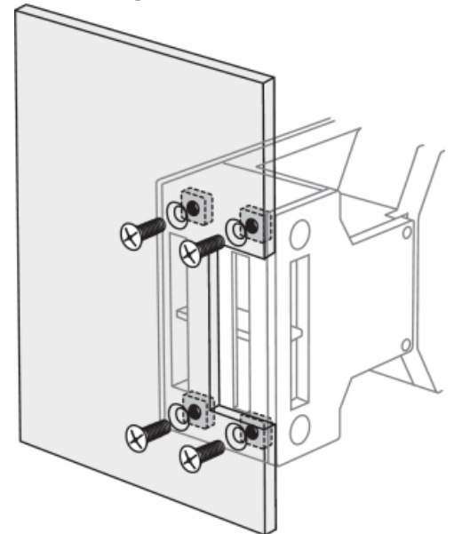
Frontmontage
