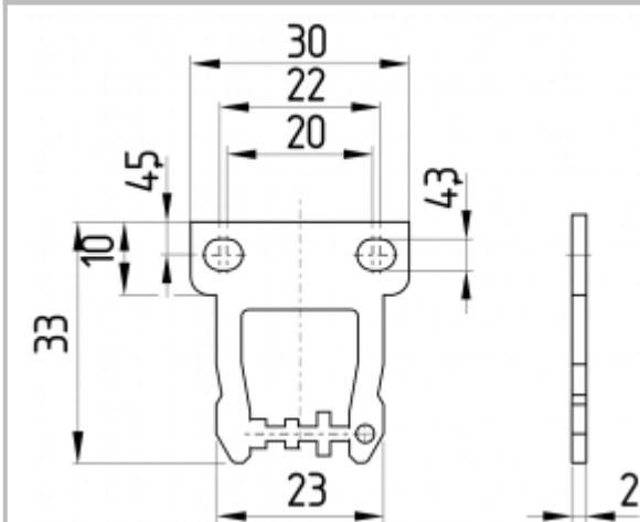
Gerader Betätiger B1
