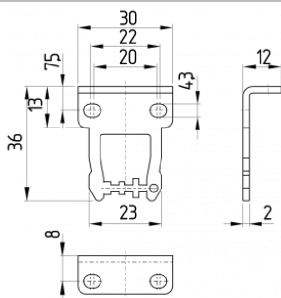
Abgewinkelter Betätiger B5
