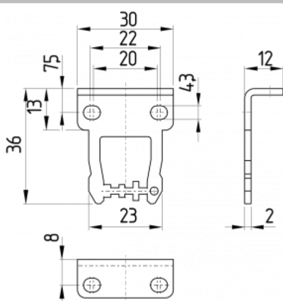
Abgewinkelter Betätiger B5
