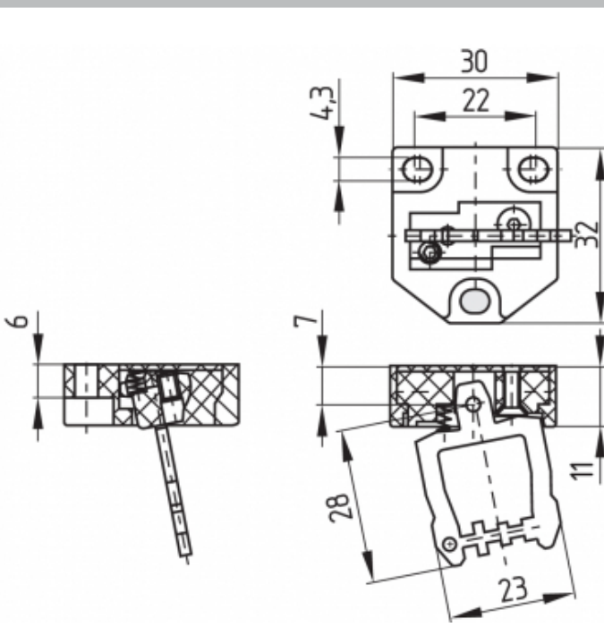
Beweglicher Betätiger B6R
