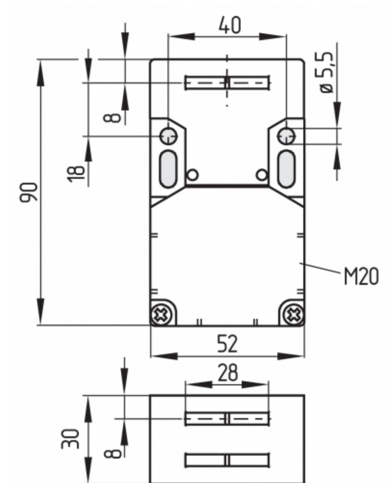
Frontmontage
