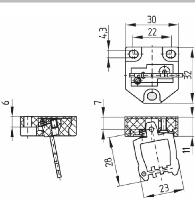
Beweglicher Betätiger B6R
