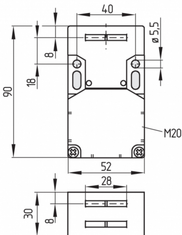
Montaje frontal
