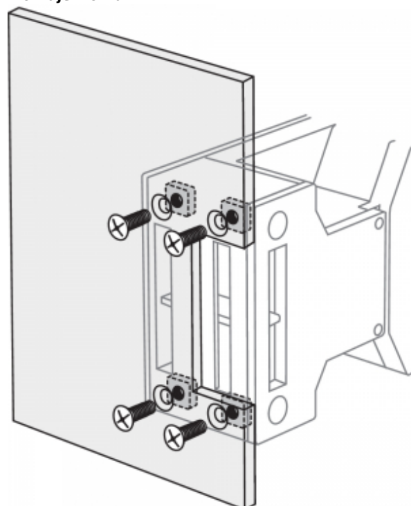
Montaje frontal
