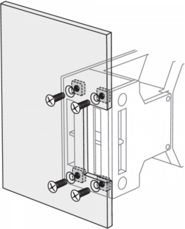
Montaje frontal
