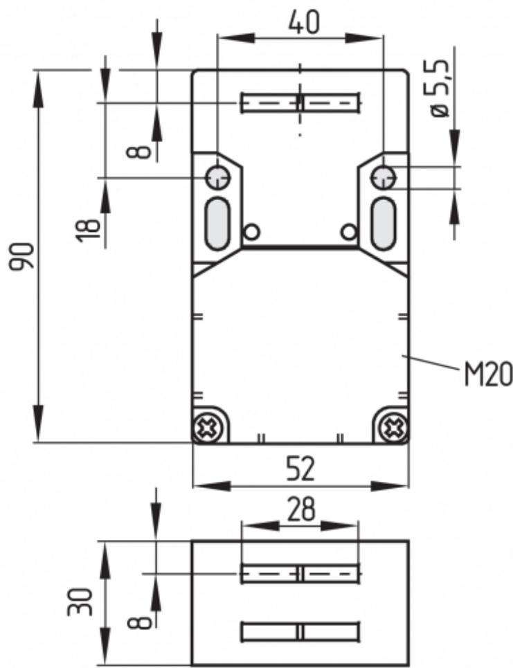
Montaje frontal
