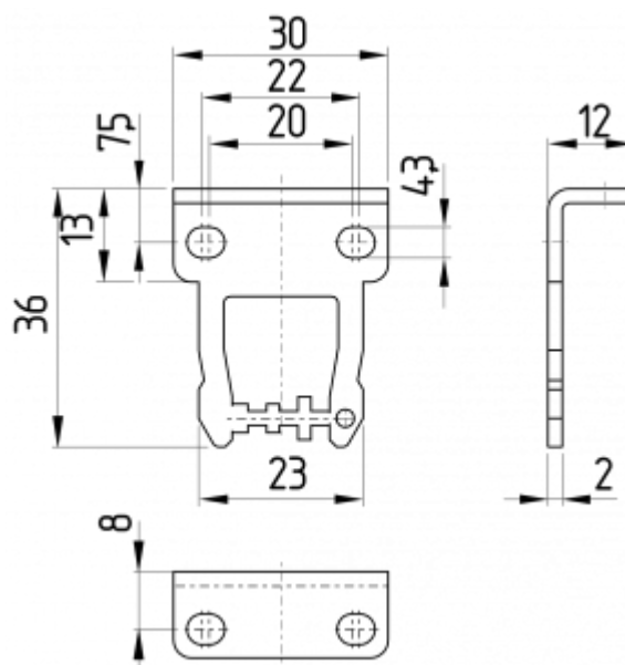
Angled actuator B5
