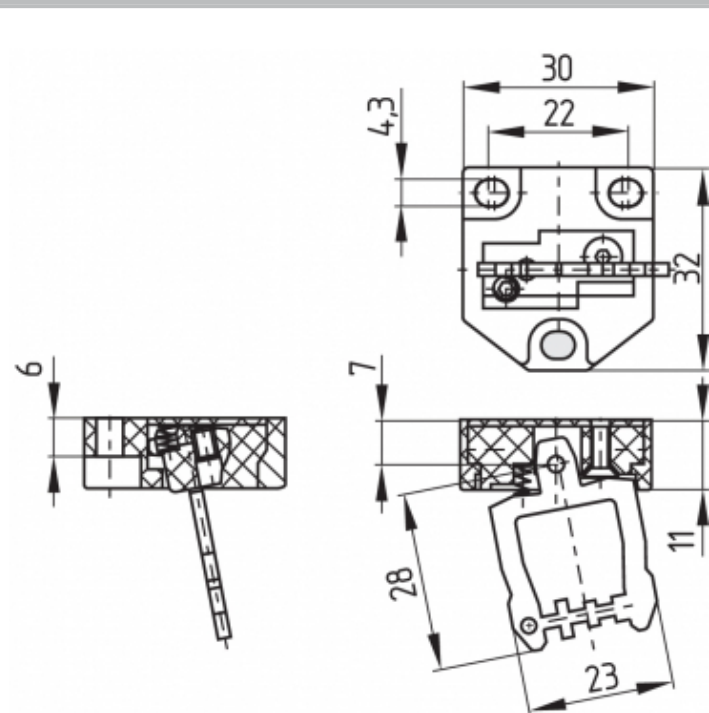
Actionneur articulé B6R
