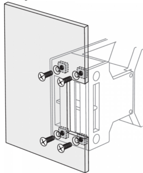
Montage frontal
