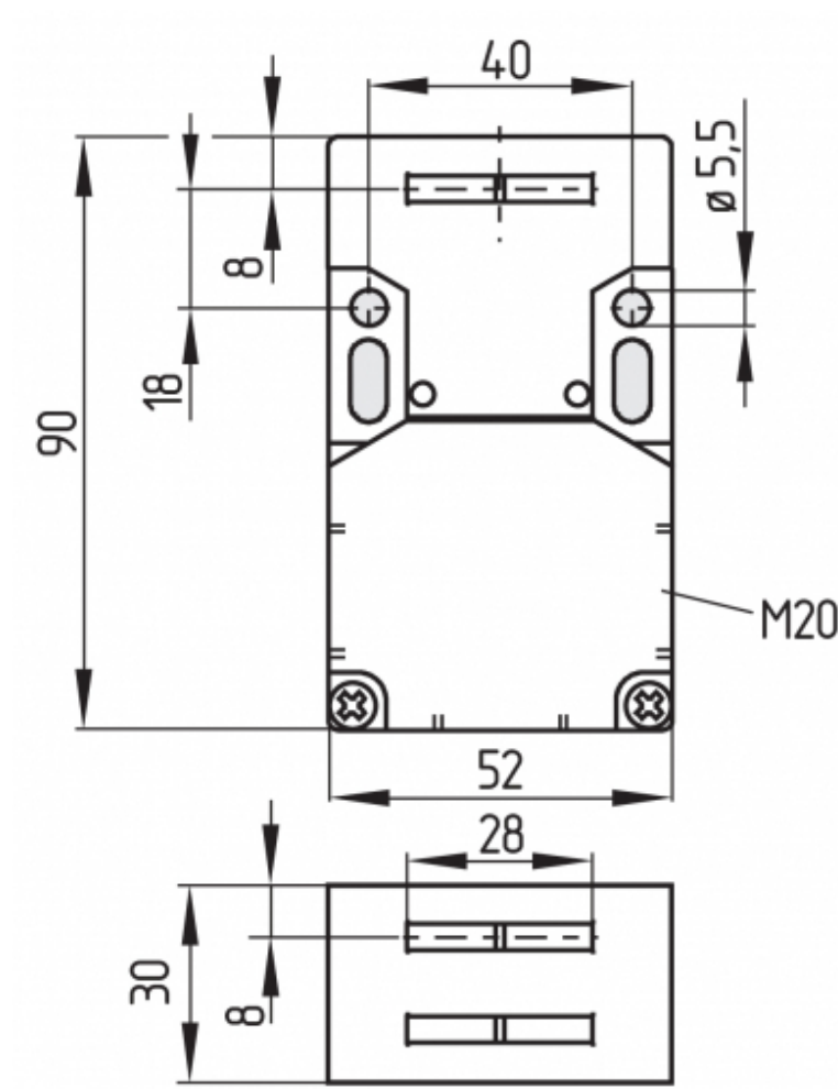
Montage frontal
