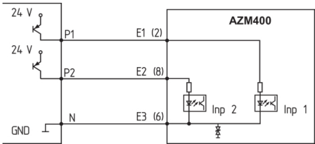
Utilisation des sorties de sécurité du type P/P: Système de commande de sécurité
