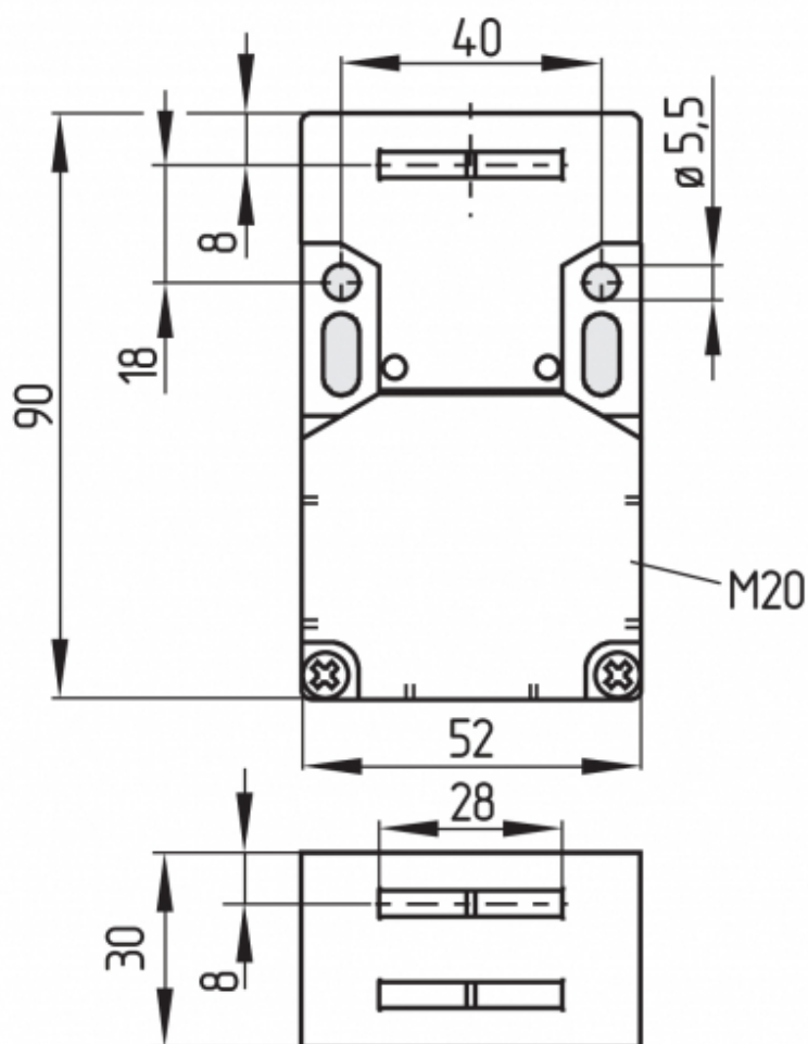
Montaggio frontale
