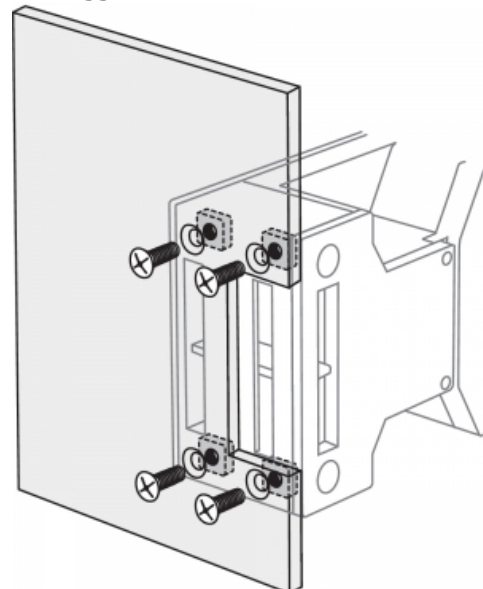
Montaggio frontale
