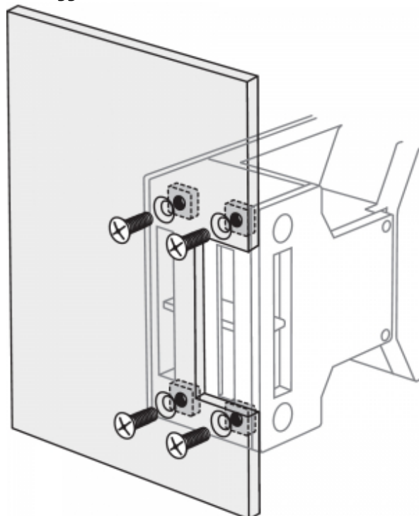
Montaggio frontale
