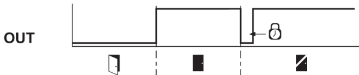
ドアロック時の通常シーケンス
