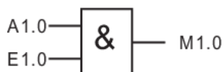
スプリングロック：IN = 0 = Lock
