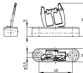
Atuador B1-2053 com retenção por esfera
