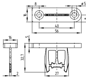
Atuador reto B1E
