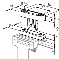
Atuador B1-2177 com auxílio de centragem
