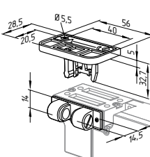
Atuador B1-2053 com retenção por esfera
