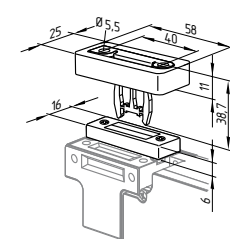
Atuador móvel B6L
