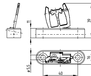
Atuador B1-2177 com auxílio de centragem
