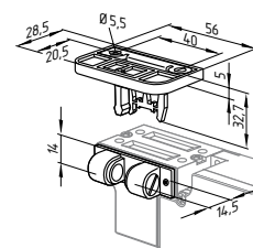
Atuador B1-1747 com íman de fixação
