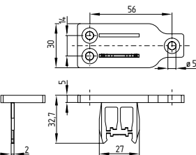
Atuador móvel B6R
