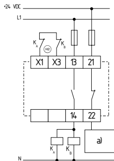
Abb. 18 a) Steuerung ⊖ = Rückführkreis
