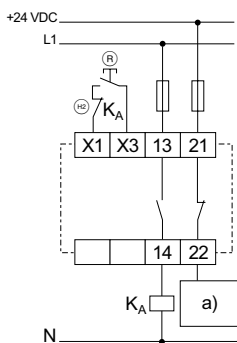
Abb. 17 a) Steuerung Ⓡ = Reset-Taster Ⓜ = Rückführkreis
