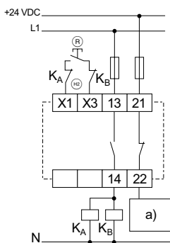
Abb. 18 a) Steuerung Ⓡ = Reset-Taster Ⓜ = Rückführkreis
