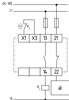
Fig. 17 a) Control ⊕ =circuito de realimentación
