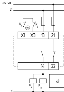
Fig. 18 a) Control ⊕ =circuito de realimentación
