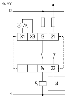
Afb. 17 a) Besturing ⊕ = Terugkoppeling
