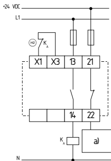
Fig. 17 a) Comando ⊖ = Circuito de retorno
