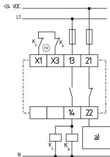
Fig. 18 a) Comando ⊖ = Circuito de retorno
