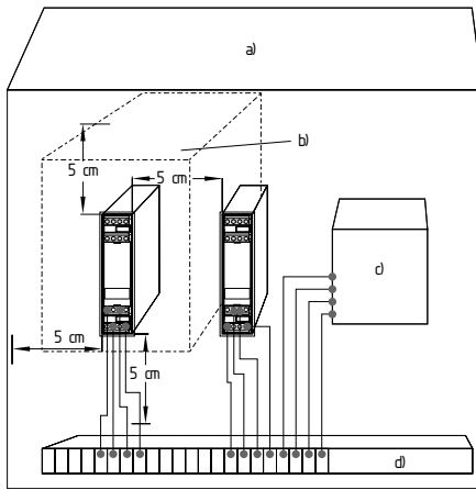
Abb. 1 a) Schaltschrank IP54 zur Installation in Zone 2 gem. EN IEC 60079-7 (ABNT NBR IEC 60079-7), EN IEC 60079-15 (ABNT NBR IEC 60079-15) geeignet b) Luft um den Baustein ca. 2.400 cm 3 (8,25 × 16 × 18,1 cm) c) Schütz (geeignet für Zone 2) d) Klemmen (geeignet für Zone 2)
