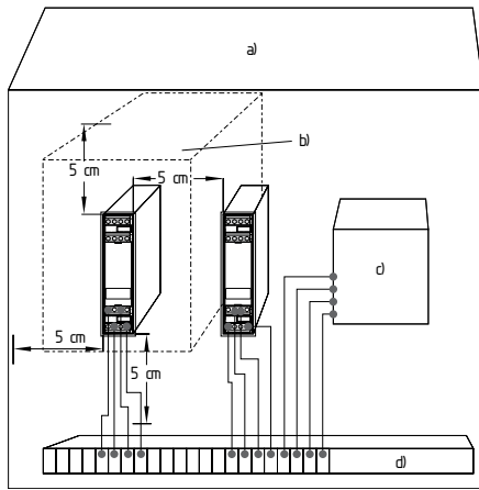
Fig. 1 a) Armario eléctrico IP54 adecuado para la instalación en la zona 2 según EN IEC 60079-7 (ABNT NBR IEC 60079-7), EN IEC 60079-15 (ABNT NBR IEC 60079-15) b) Espacio libre alrededor del relé aprox. 2.400 cm 3 (8,25 × 16 × 18,1 cm) c) Contactor (adecuado para zona 2) d) Bornes (adecuados para zona 2)
