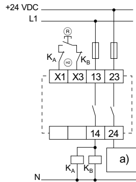
Fig. 18 a) Control Ⓡ = pulsador de rearme Ⓢ = circuito de realimentación
