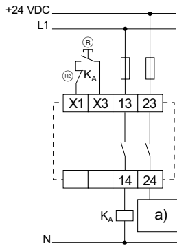
Fig. 17 a) Control Ⓡ = pulsador de rearme Ⓢ = circuito de realimentación
