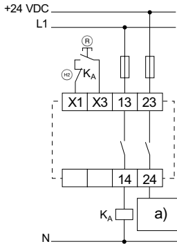
Fig. 17 a) Controllo Ⓜ = pulsante di Reset Ⓜ = circuito di ripristino
