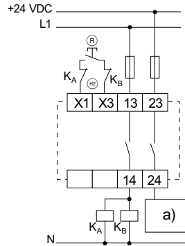
Fig. 18 a) Controllo Ⓜ = pulsante di Reset Ⓜ = circuito di ripristino
