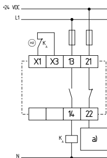
Afb. 17 a) Besturing ⊖ = Terugkoppeling
