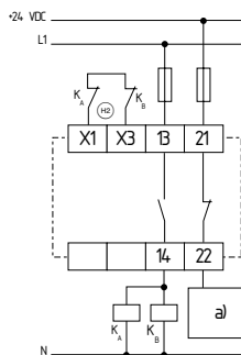
Afb. 18 a) Besturing ⊖ = Terugkoppeling
