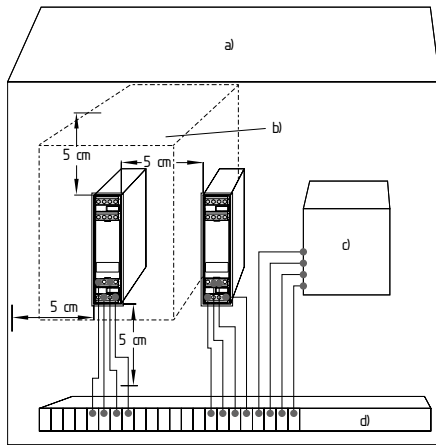
Fig. 1 a) Caixa de comutação IP54 adequada para instalação na zona 2, de acordo com EN IEC 60079-7 (ABNT NBR IEC 60079-7), EN IEC 60079-15 (ABNT NBR IEC 60079-15) b) Ar em torno do módulo aprox. 2.400 cm 3 (8,25 × 16 × 18,1 cm) c) Contator (adequado para a zona 2) d) Terminais (adequados para a zona 2)
