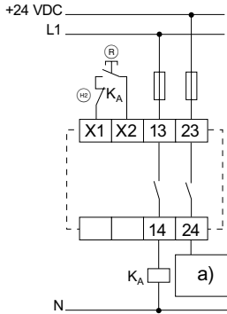
Abb. 16 a) Steuerung Ⓡ = Reset-Taster Ⓜ = Rückführkreis
