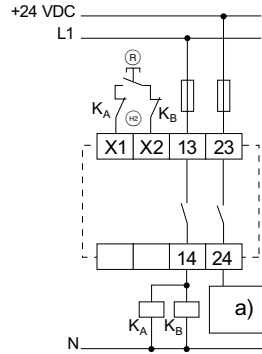
Abb. 17 a) Steuerung Ⓡ = Reset-Taster Ⓜ = Rückführkreis
