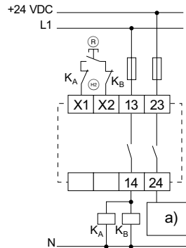
Fig. 17 a) Bloc logique Ⓡ = Bouton de réarmement Ⓢ = Boucle de retour
