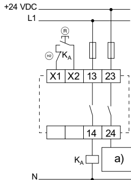
Fig. 16 a) Bloc logique Ⓡ = Bouton de réarmement Ⓢ = Boucle de retour
