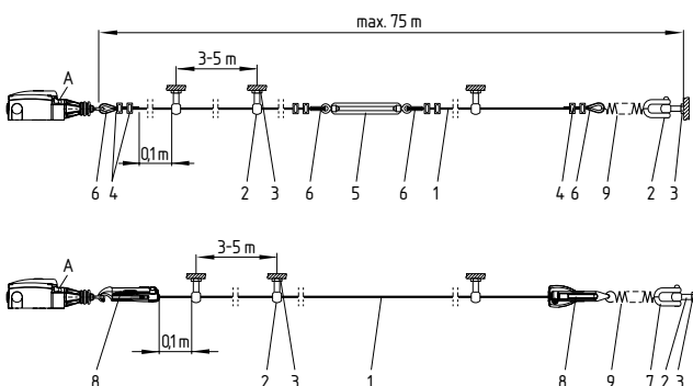
Rys. 2: Montaż komponentów
