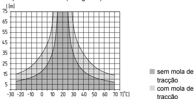
Figura 3: comprimento máximo do cabo dependendo da temperatura, com ou sem mola de tracção
