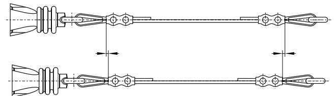
Afbeelding 4: vervorming van de kabelkousen
