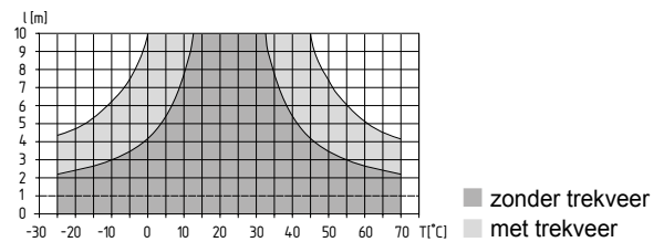
Afbeelding 3: Maximale kabel lengte in functie van de temperatuur met of zonder trekveer
