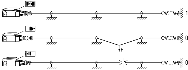
Image 1: indicateur de position et d'actionnement
