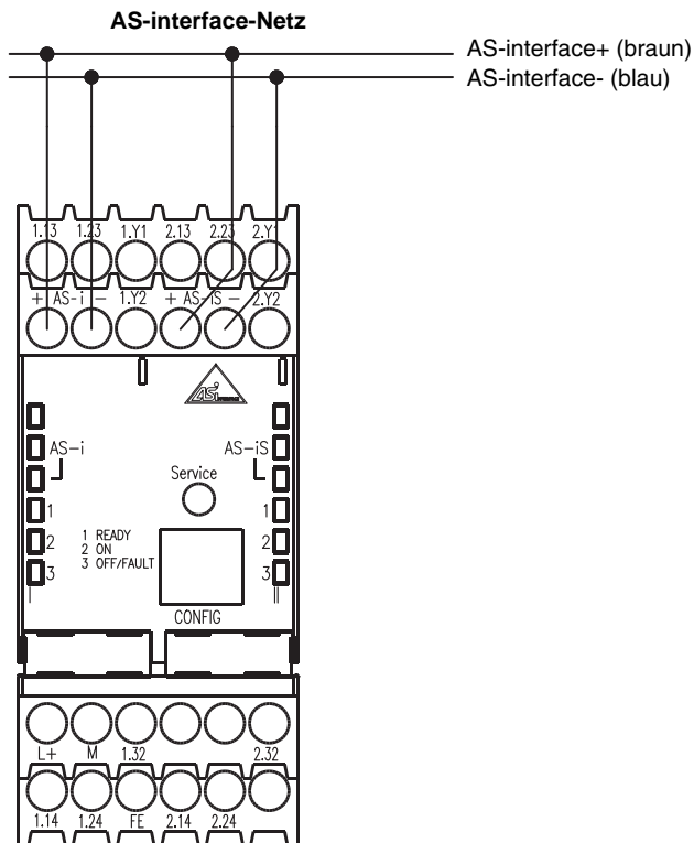
Bild 7.3: Anschluss der Klemmen des sicheren AS-interface-Ausgangs zur Aktor-Überwachung
