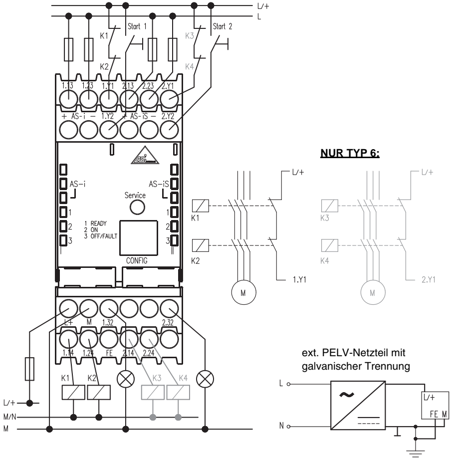
Bild 7.2: Anschlussübersicht AS-interface-Sicherheitsmonitor Typ 5 und 6
