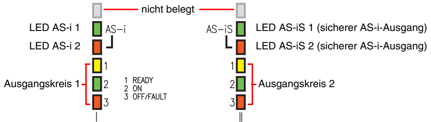
Bild 9.1: Übersicht Geräte-LEDs
