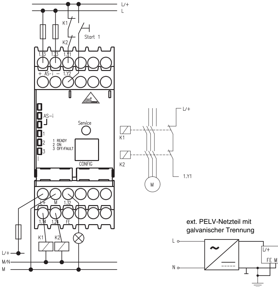
Bild 5.2: Anschlussübersicht AS-interface-Sicherheitsmonitor Typ 1 und 3
