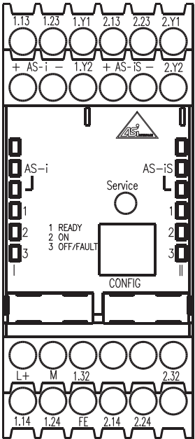
Bild 7.1: Klemmenanordnung / Blockschaltbild AS-interface-Sicherheitsmonitor Typ 5 und 6
