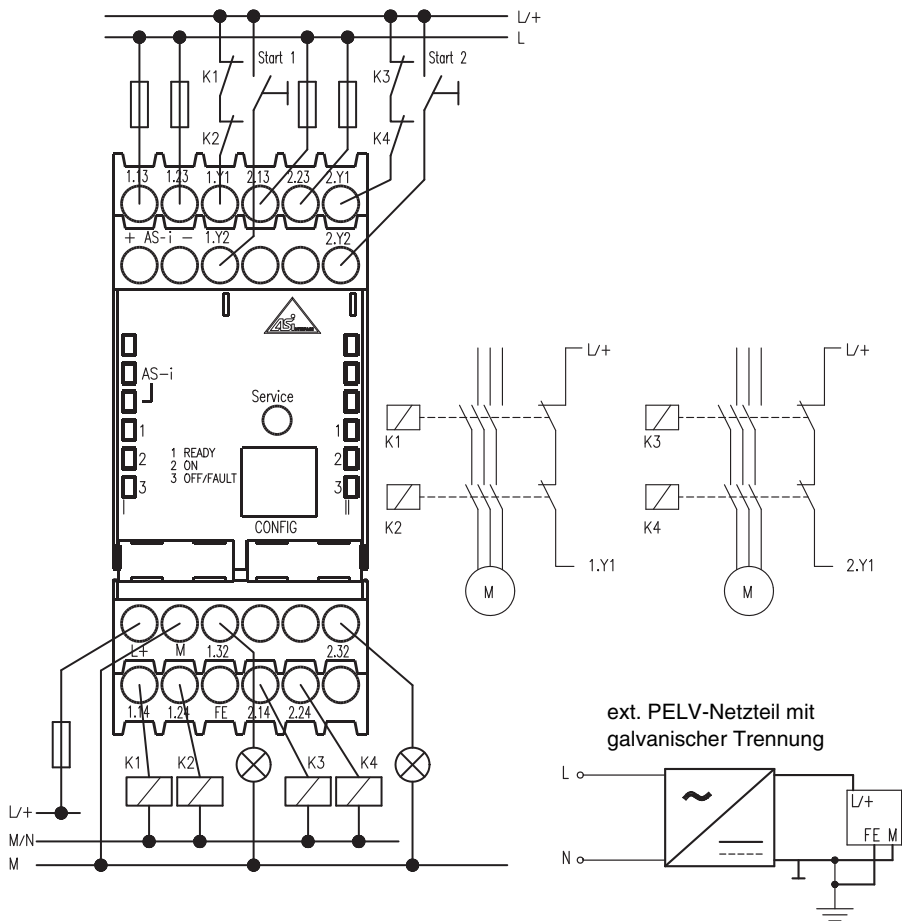
Bild 6.2: Anschlussübersicht AS-interface-Sicherheitsmonitor Typ 2 und 4
