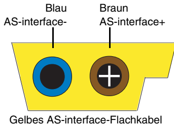
Bild 8.1: AS-interface-Kabelvarianten
