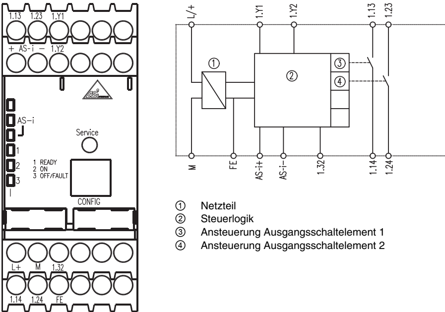
Bild 5.1: Klemmenanordnung / Blockschaltbild AS-interface-Sicherheitsmonitor Typ 1 und 3
