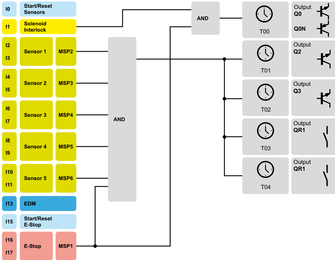
Diagrama de funciones del programa de aplicación 3
