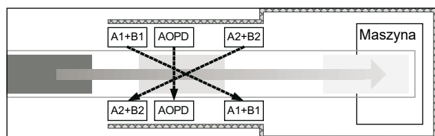
Muting z 2 czujnikami
