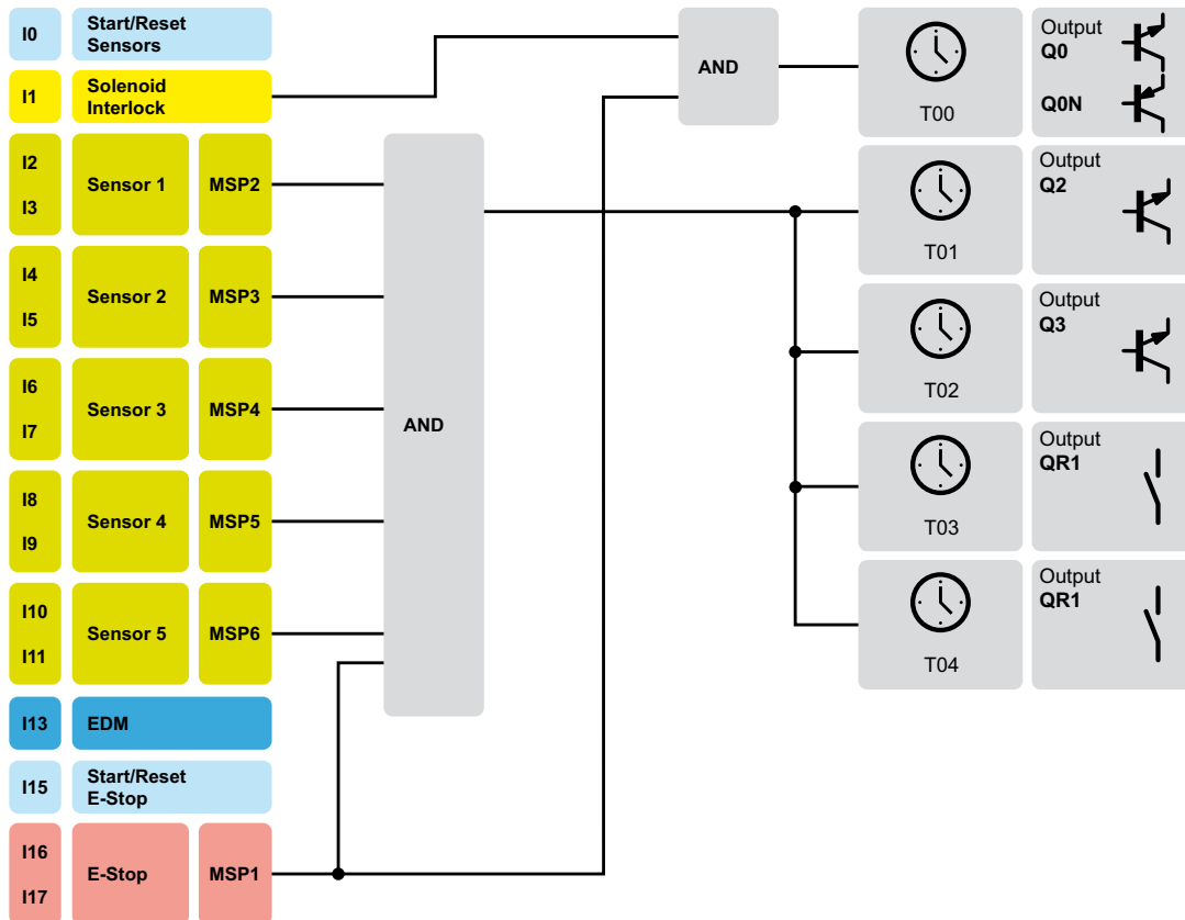
Schemat funkcji programu aplikacyjnego 3
