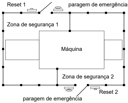
Esquema programa de aplicação 2
