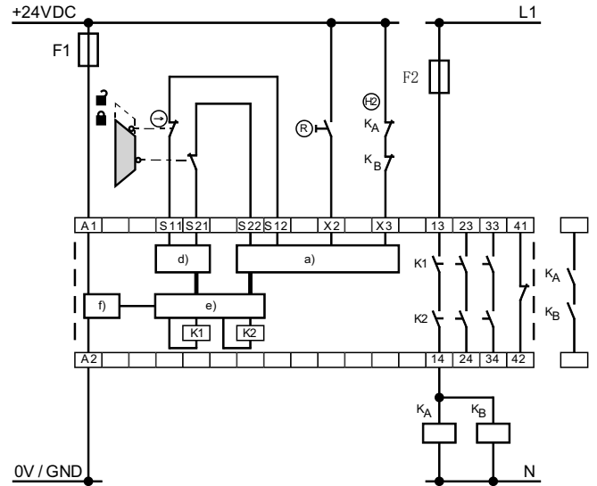
接线图示 SRB-E-301ST
