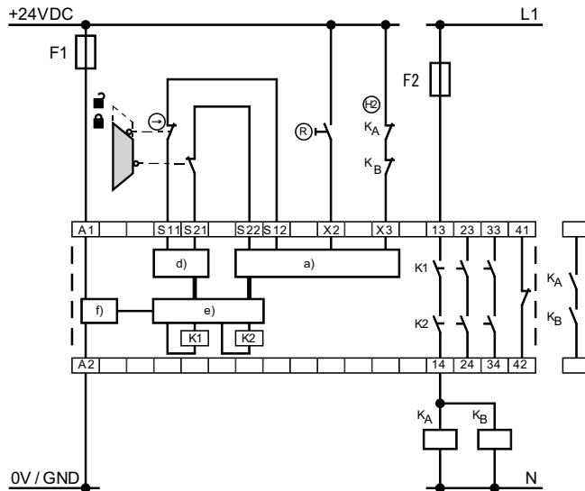
SRB-E-301STの配線例
