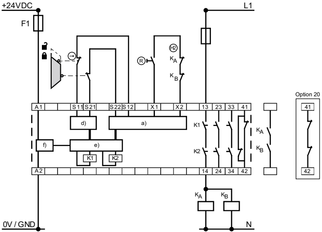
配線例
