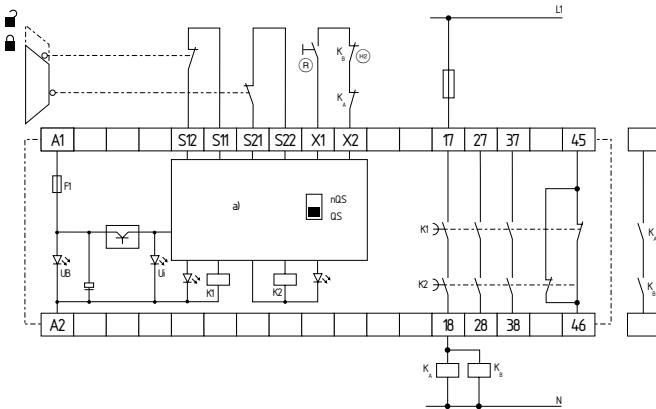
Afb. 4 a) Besturing
