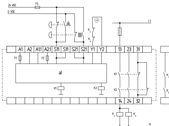
Fig. 2 a) Lógica de comando
