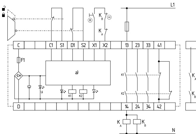
Fig. 2 a) Lógica de control Ⓜ = circuito de realimentación
