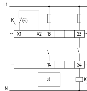
Fig. 9 a) Habilidad del regulador
