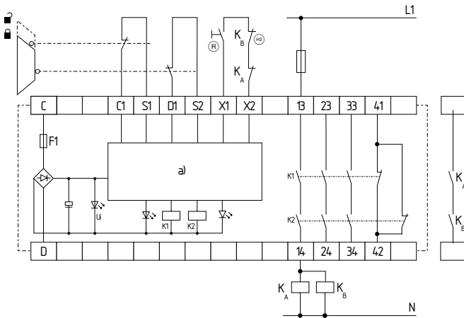
図2 a) 制御ロジック Ⓡ = バックチェック回路
