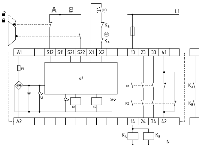
Fig. 2 a) Lógica de control ⊕ = circuito de realimentación
