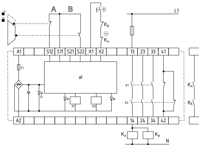
Fig. 2 a) Bloc logique ® = Boucle de retour
